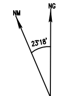
Declinação Magnética
