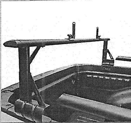
SUORTE DE ESCADA PARA CAÇAMBA 50928986
